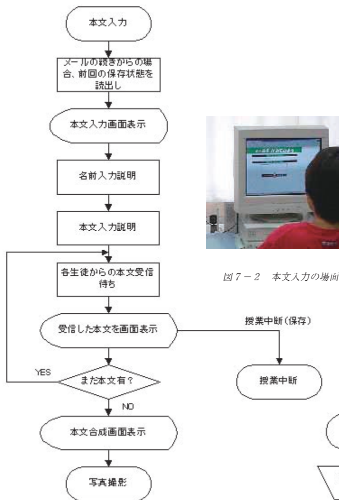
図7-1 メール本文入力部のフローチャート
