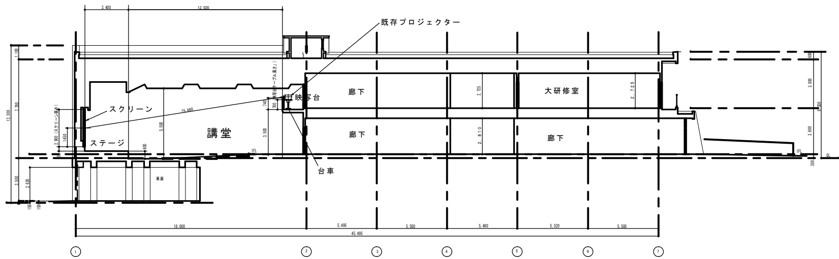
断面図 1/100
