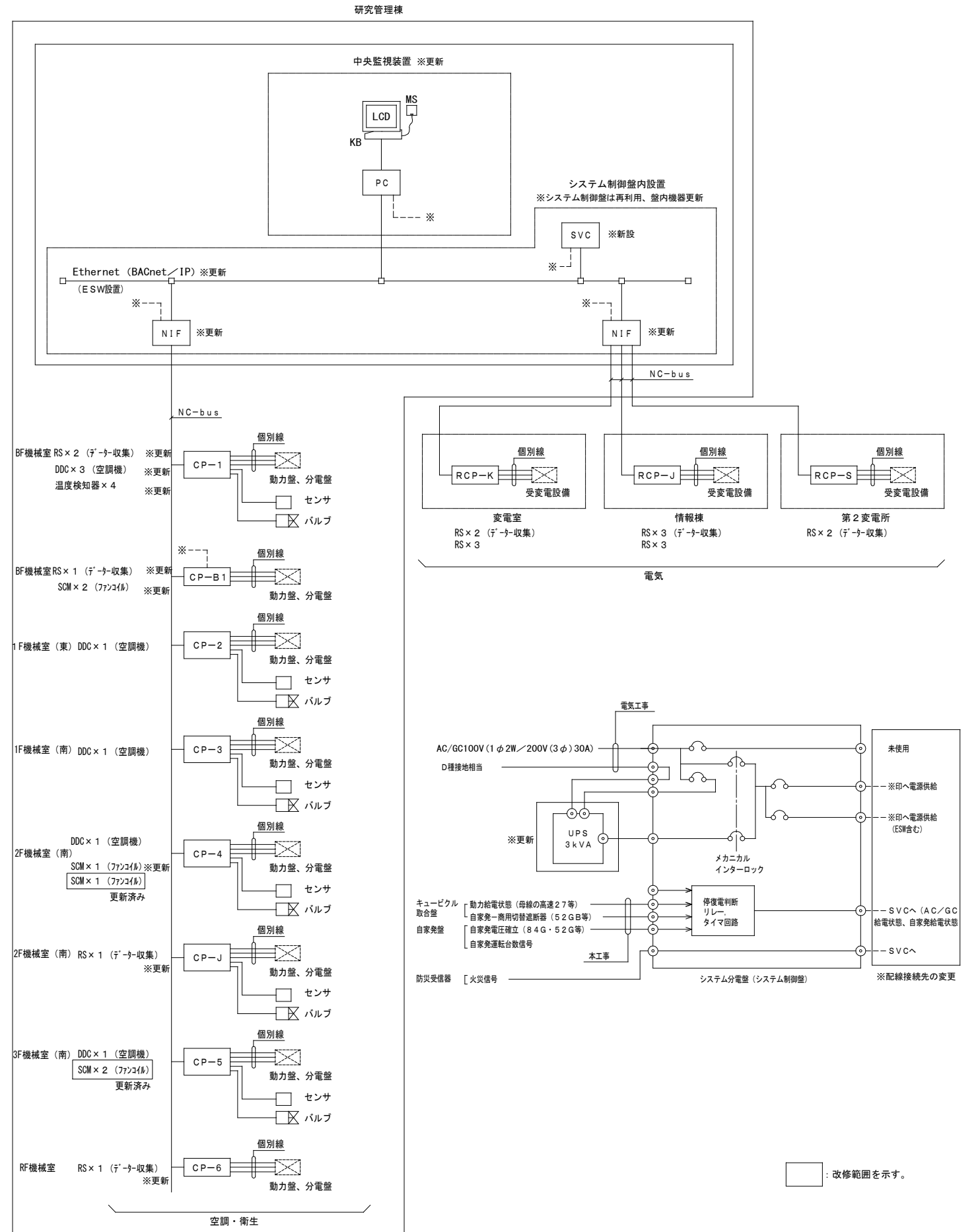
システム構成図（改修後）
