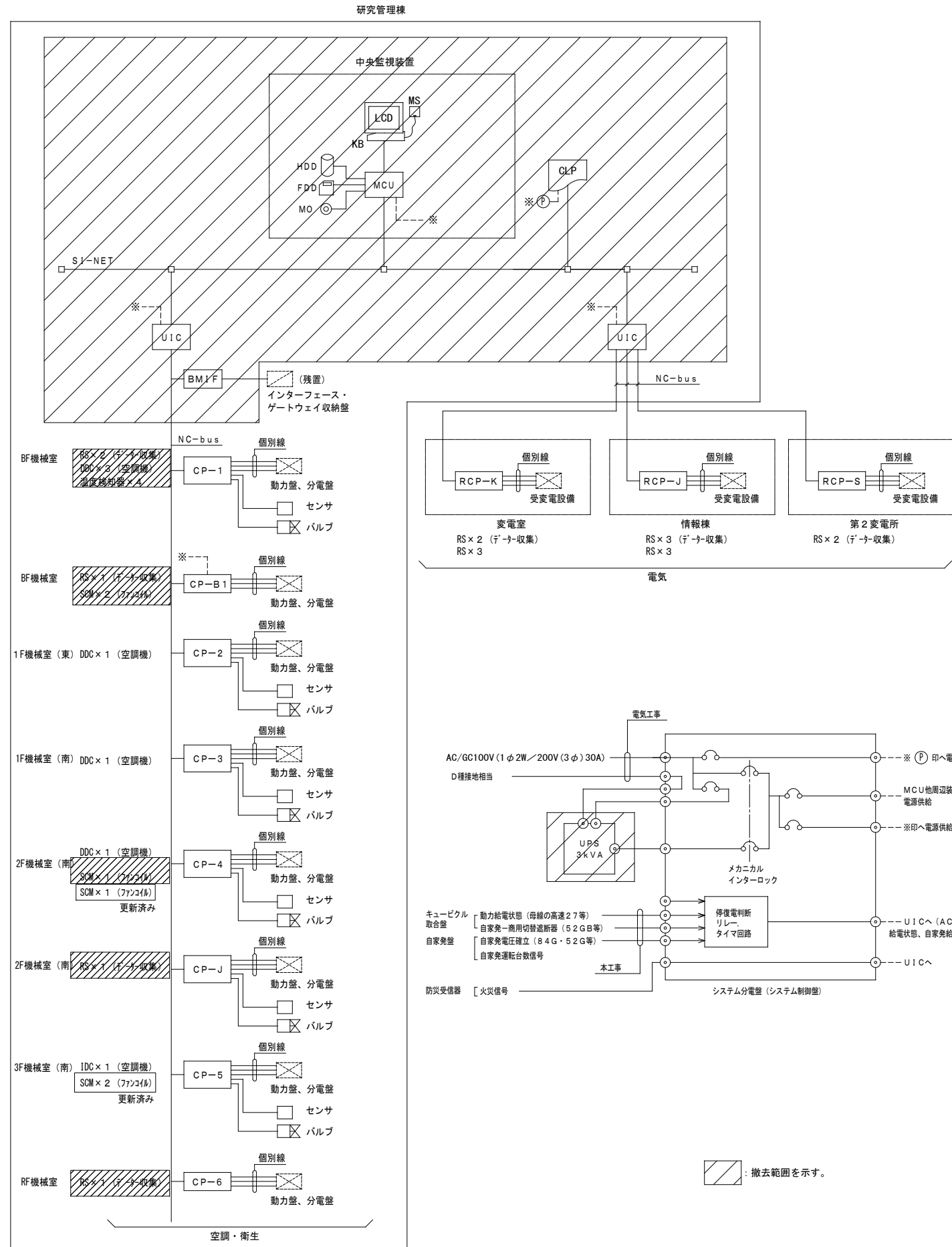
システム構成図（改修前）
